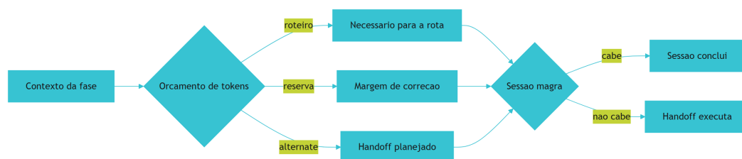
Figura 10: Orçamento de contexto de uma sessão agêntica
