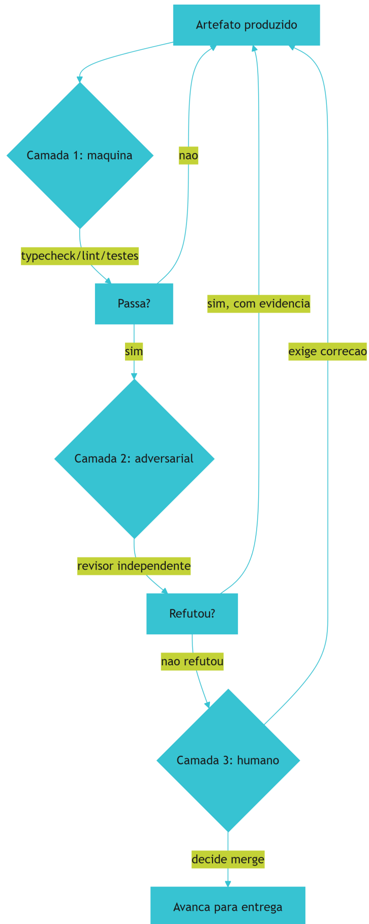
Figura 6: Três camadas de verificação adversarial com evidência
